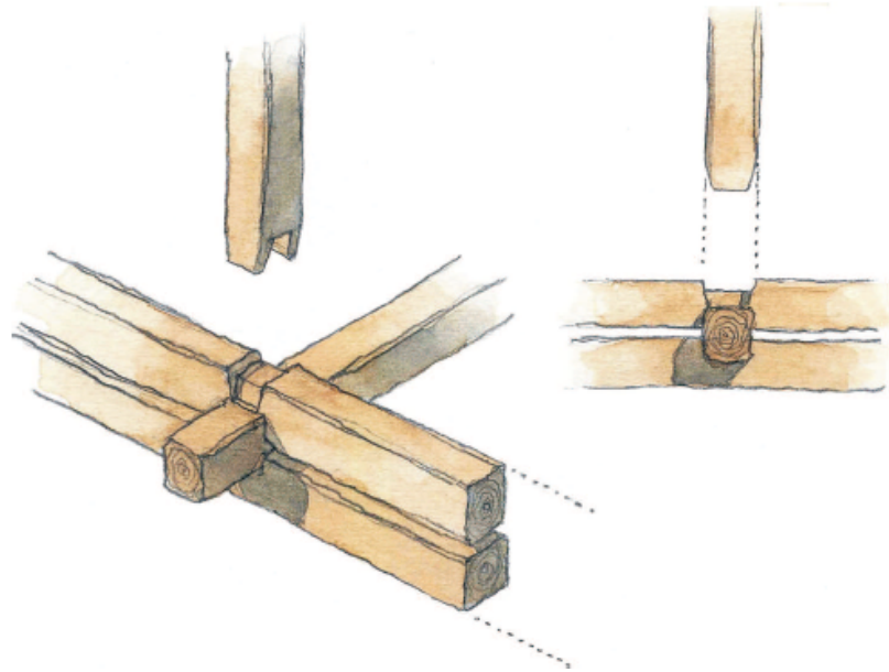
C - pilastro centrale / travi di base
