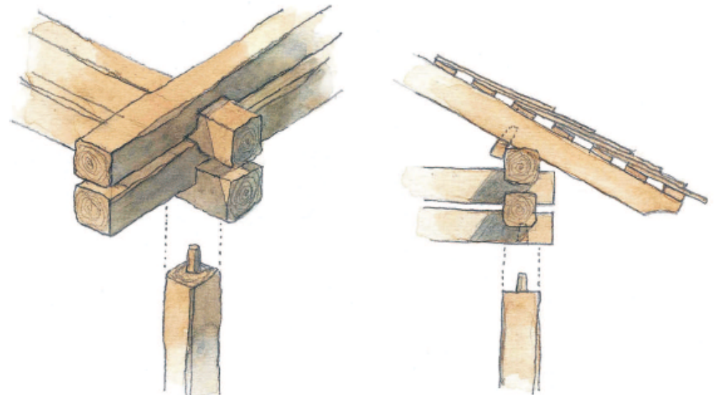
A - pilastro d'angolo / banchine
