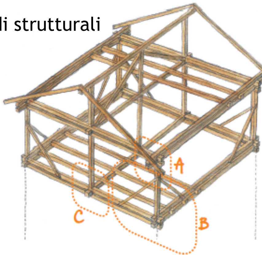
C - pilastro centrale / travi di base
